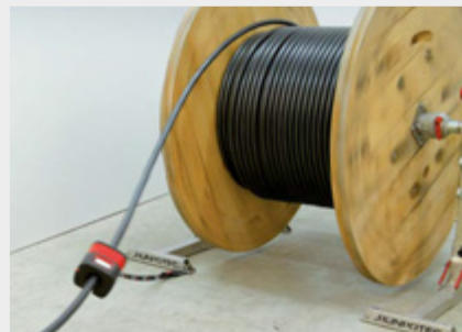
RM35 mit RUNPOLIFTER L1600 und 3 x 35 mm² Kabel
